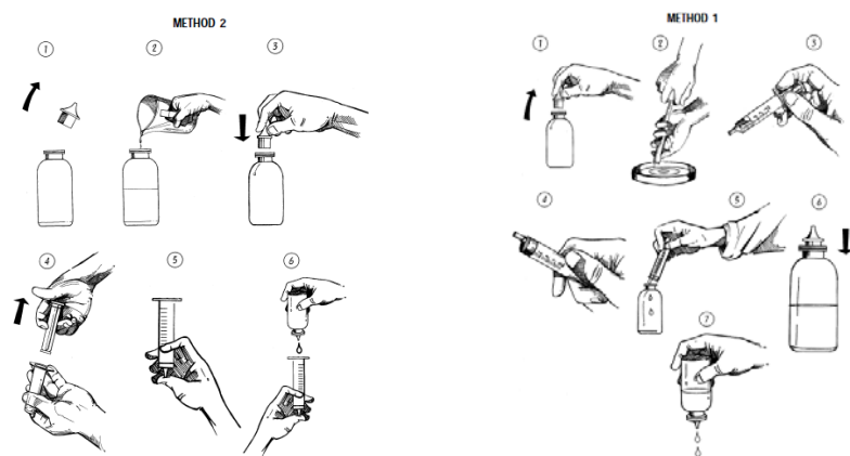
شکل ۱۴- نحوه آزمایش صحت عملکرد قطره چکان
